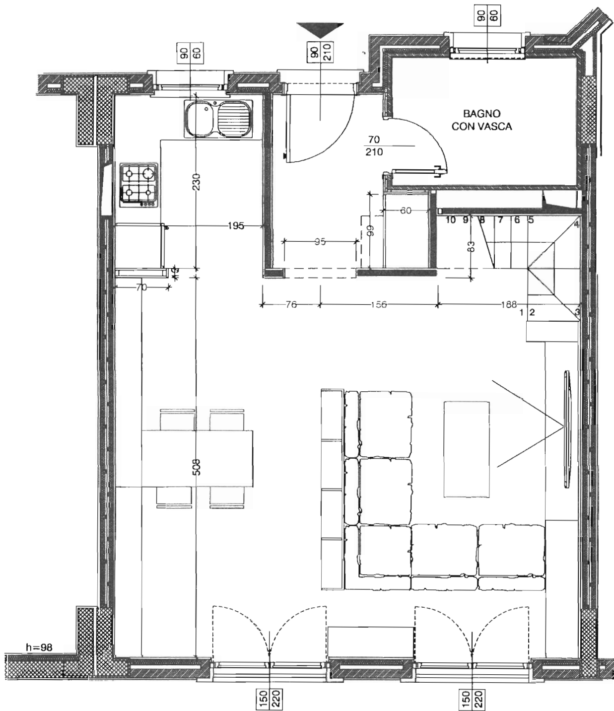
DUPLEX : piano 1° - scala 1 : 50
