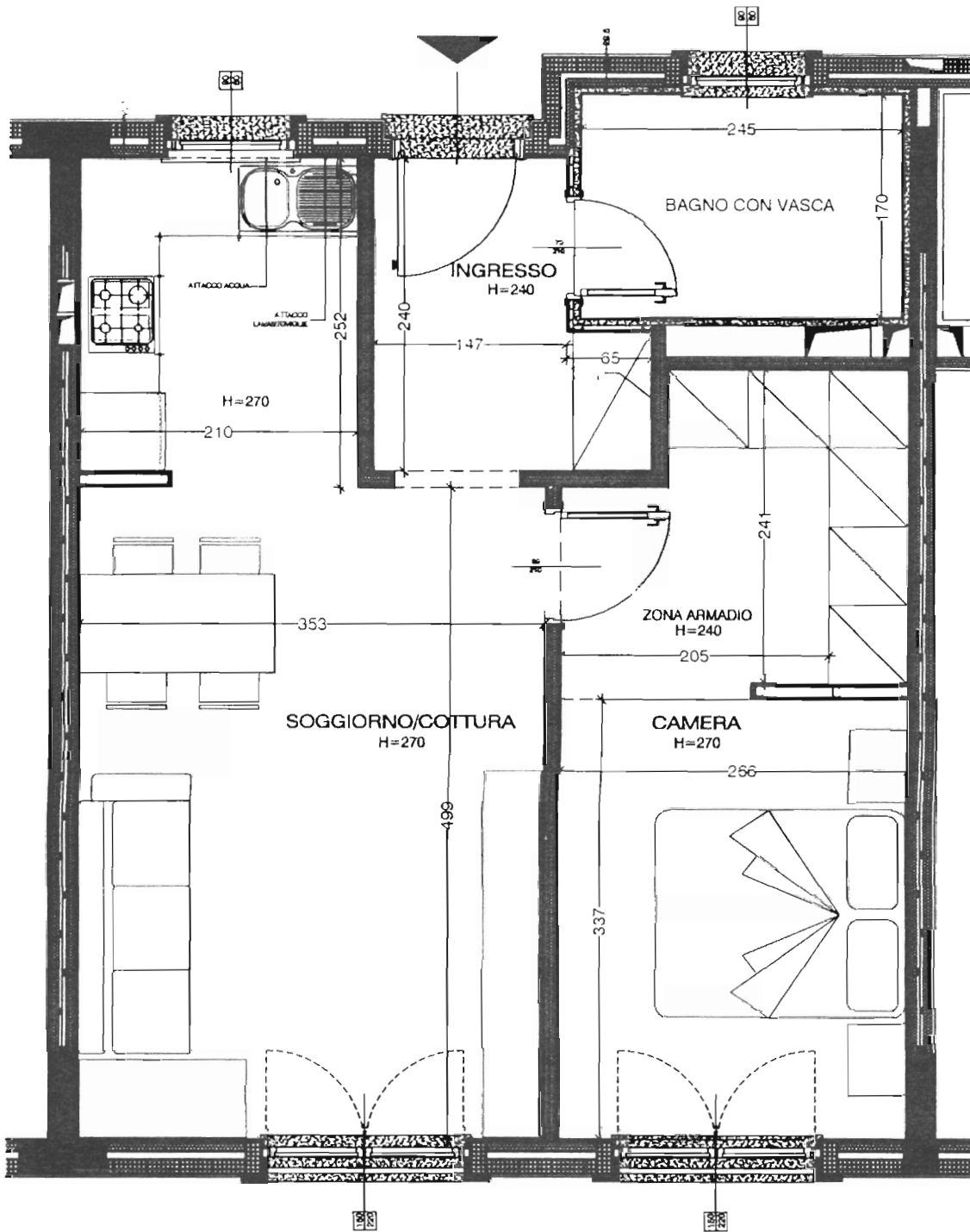
BILOCALE TIPO - scala 1 : 50
